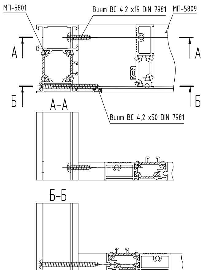
Узел крепления порга МП-5809 к раме МП-5801
